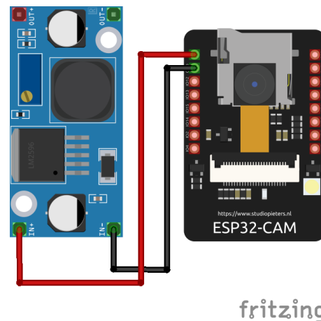
Gambar 4. Perancangan sumber daya untuk esp32 cam
