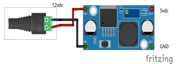
Gambar 3. Perancangan Sumber Daya
