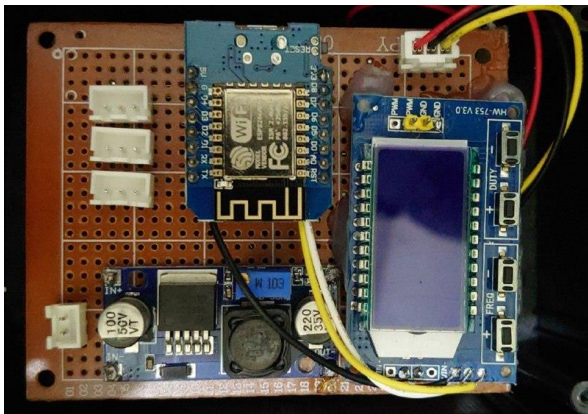
Gambar 9. Alat Pembangkit Suara Ultrasonik
